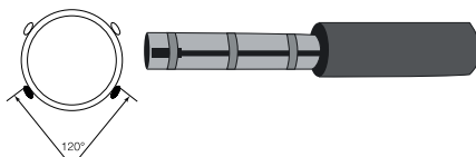
Установка кабеля в позиции 4 и 8 часов
